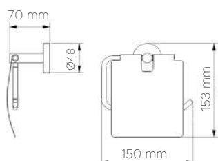
TECHNICAL DETAILS DONNÉES TECHNIQUES 05154
