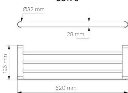
TECHNICAL DETAILS DONNÉES TECHNIQUES 05176
