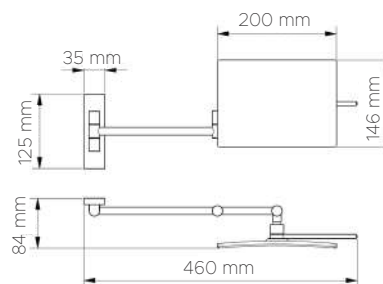
TECHNICAL DETAILS DONNÉES TECHNIQUES 05163 • 05183
