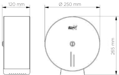
TECHNICAL DETAILS DONNÉES TECHNIQUES 06004 • 06005 • 06054 • 06056
