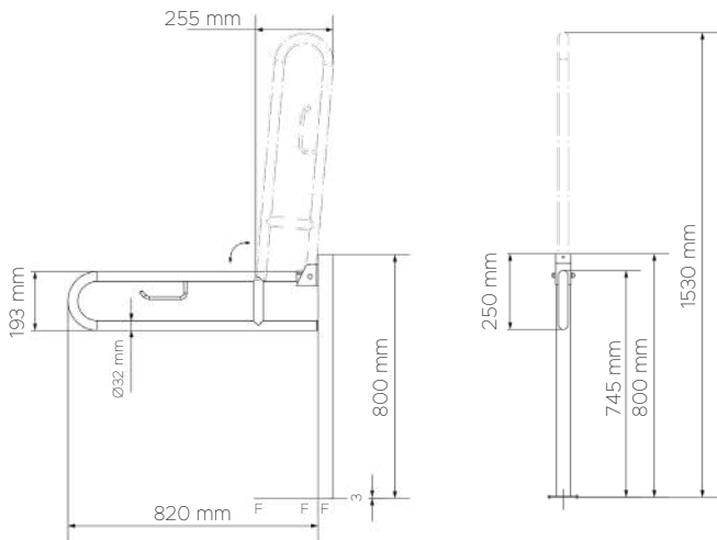
TECHNICAL DETAILS DONNÉES TECHNIQUES 02004 • 02033 • 02110
