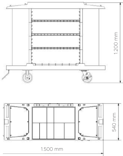
TECHNICAL DETAILS DONNÉES TECHNIQUES 08017
