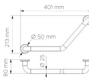
TECHNICAL DETAILS DONNÉES TECHNIQUES 05097
