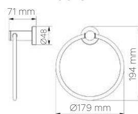
TECHNICAL DETAILS DONNÉES TECHNIQUES 05152
