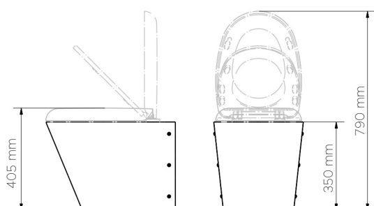
TECHNICAL DETAILS DONNÉES TECHNIQUES 03014 • 03015
