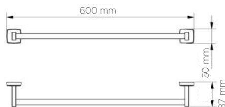
TECHNICAL DETAILS DONNÉES TECHNIQUES 05066 • 05067
