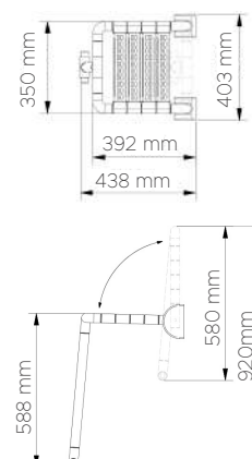
TECHNICAL DETAILS DONNÉES TECHNIQUES 02083
