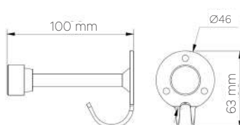
TECHNICAL DETAILS DONNÉES TECHNIQUES 05080
