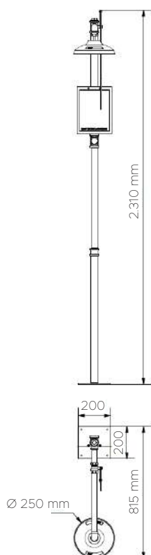
TECHNICAL DETAILS DONNÉES TECHNIQUES 12023
