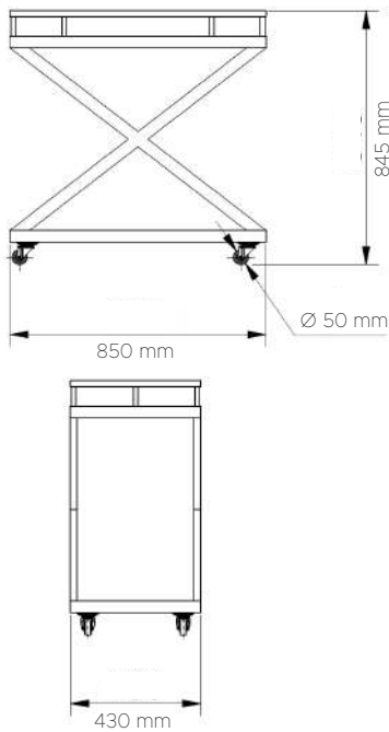
TECHNICAL DETAILS DONNÉES TECHNIQUES 08058
