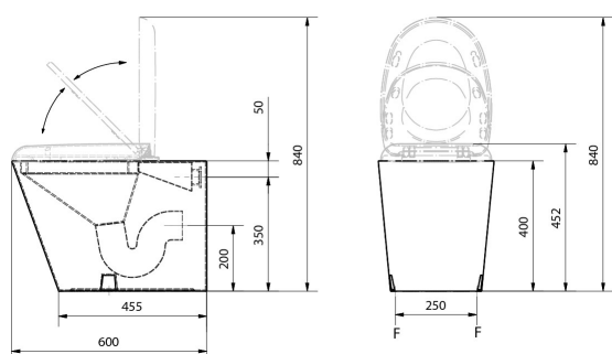
TECHNICAL DETAILS DONNÉES TECHNIQUES 03014 • 03015
