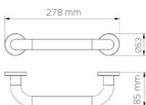
TECHNICAL DETAILS DONNÉES TECHNIQUES 05150
