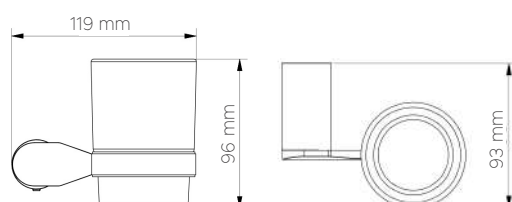
TECHNICAL DETAILS DONNÉES TECHNIQUES 05173
