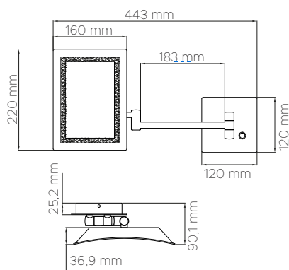
TECHNICAL DETAILS DONNÉES TECHNIQUES 05181
