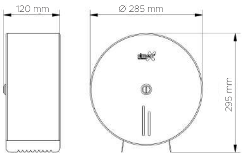
TECHNICAL DETAILS DONNÉES TECHNIQUES 06021 • 06022 • 06055 • 06068
