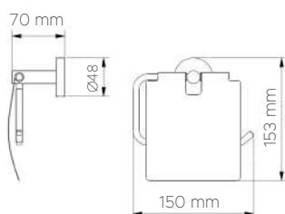
TECHNICAL DETAILS DONNÉES TECHNIQUES 05129 • 05030
