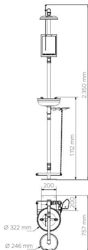
TECHNICAL DETAILS DONNÉES TECHNIQUES 12028
